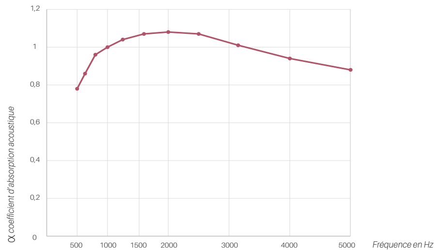
Mesures d'absorption acoustique d'un panneau Sérénity 120 x 60
