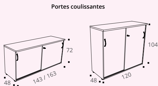
Portes coulissantes
