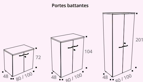
Portes battantes
