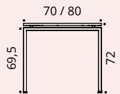
Pied arche
