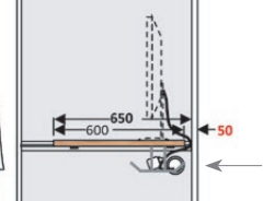
Passage pour câbles (à prévoir à la commande)
